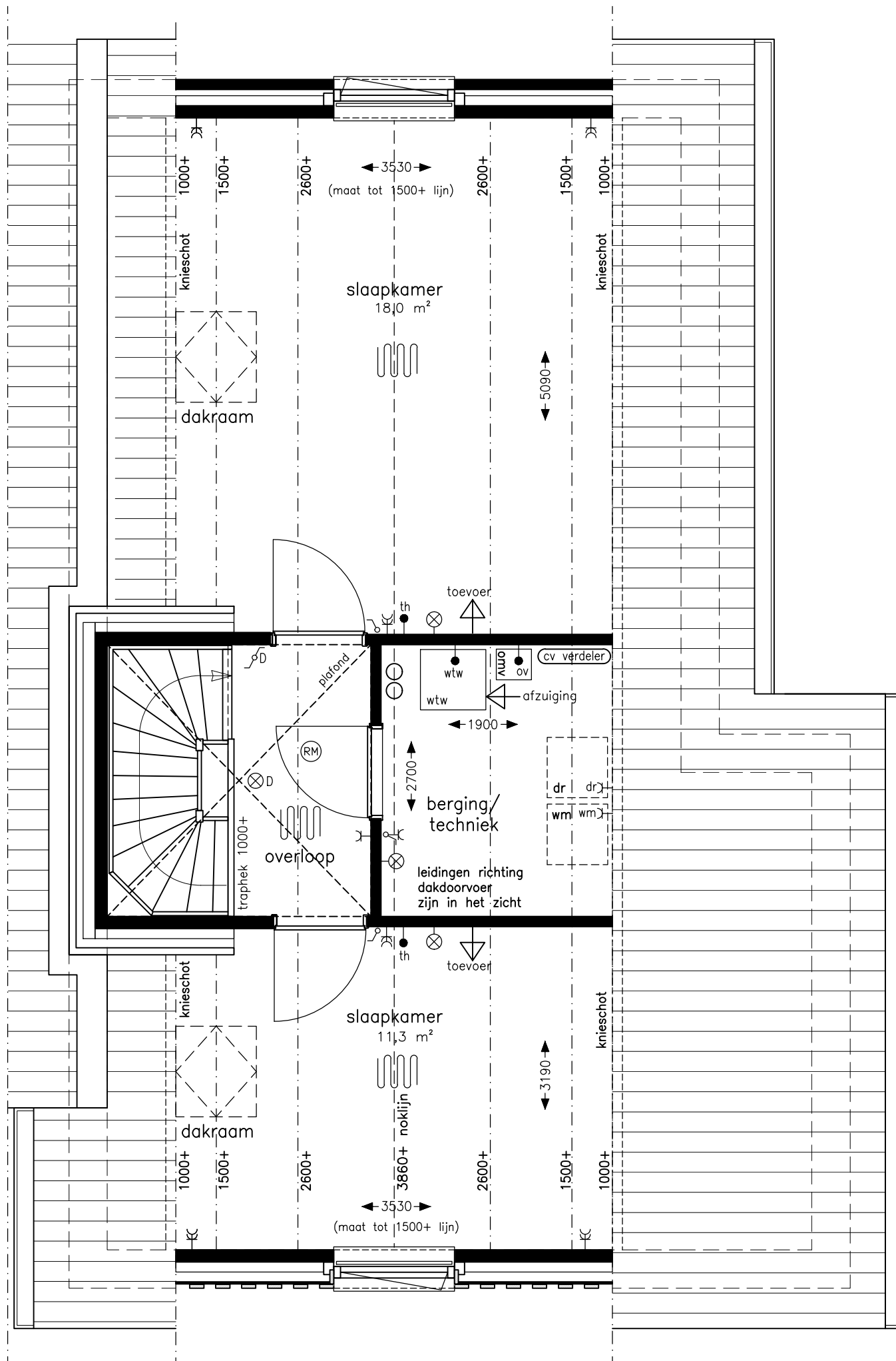
2e verdieping type B-P06 kavel indicatief schaal 1:50
