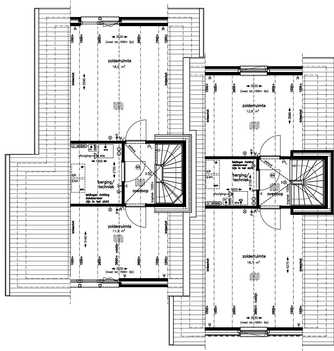
2e verdieping type B-P13 schaal 1:50
