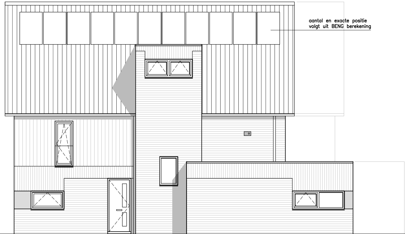
rechter zijgevel type A-P12 schaal 1:50
