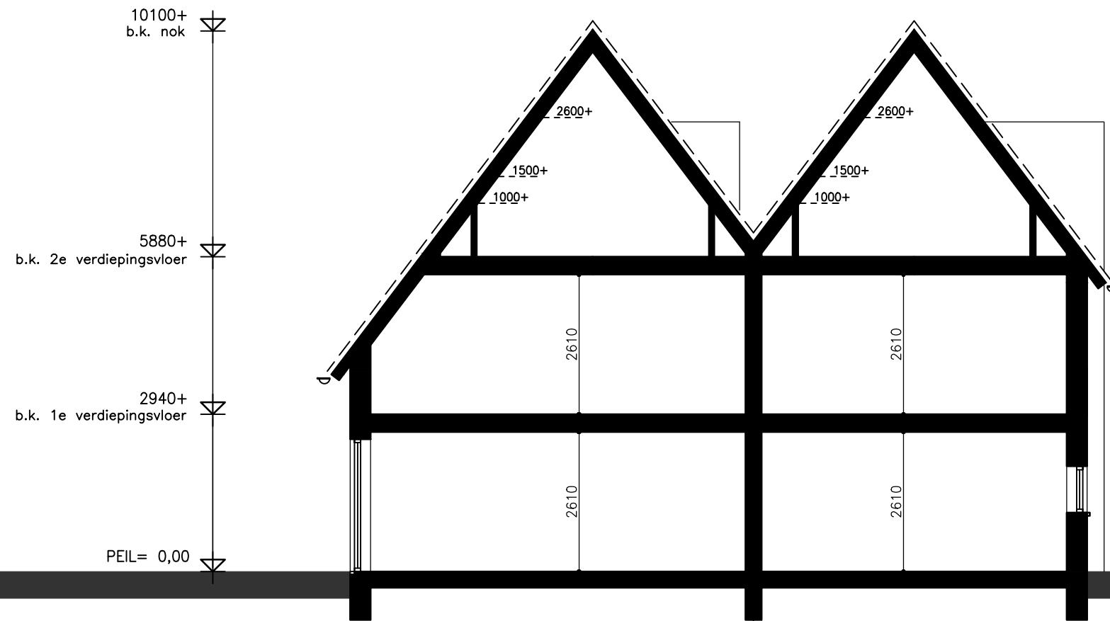
doorsnede type B-P13 schaal 1:50
