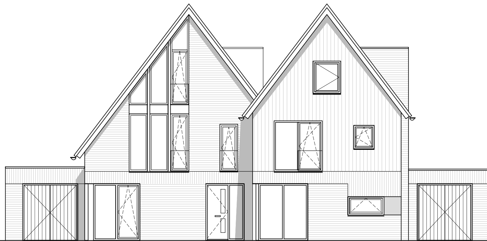
voorgevel type B-P13 schaal 1:50
