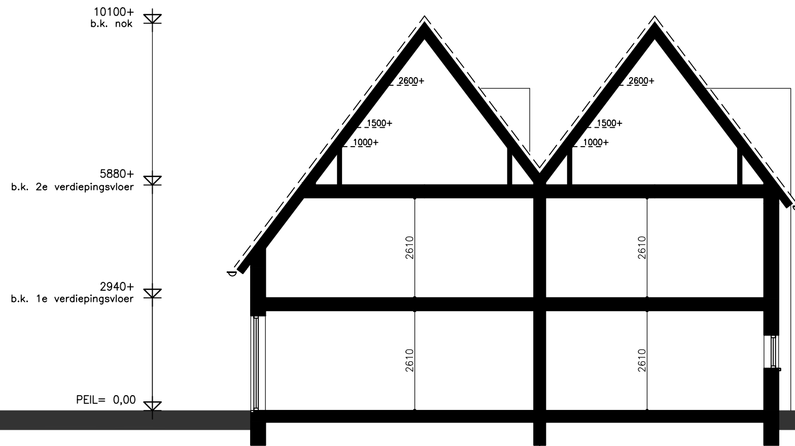
doorsnede type B-P13 schaal 1:50
