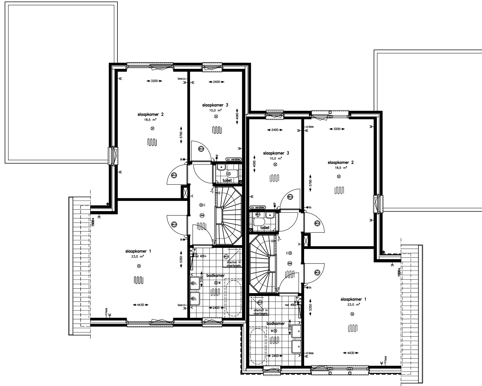
1e verdieping type B-P10 schaal 1:50
