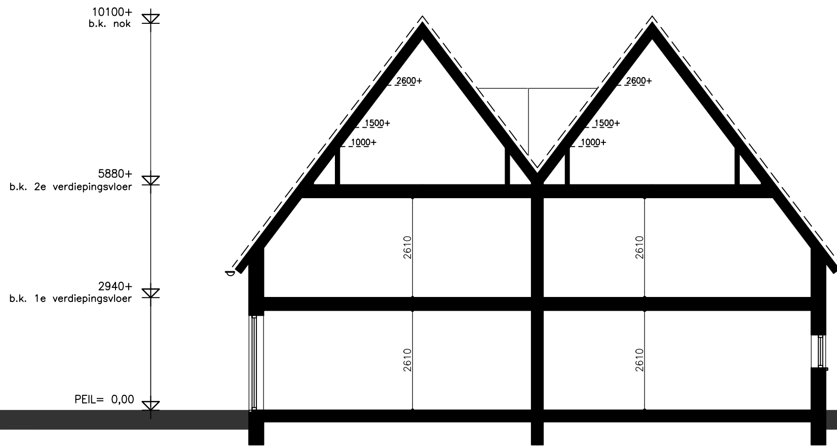
doorsnede type B-P10 schaal 1:50
