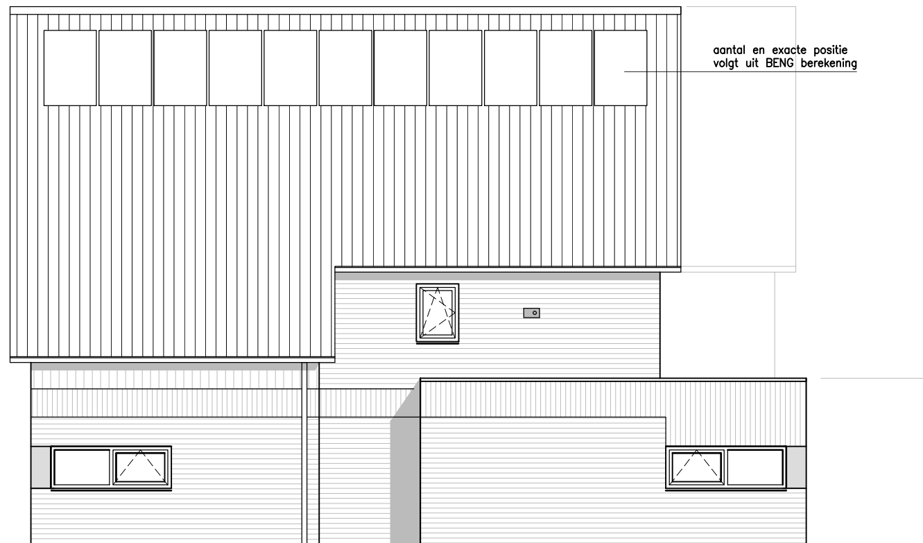
rechter zijgevel type B-P09 schaal 1:50
