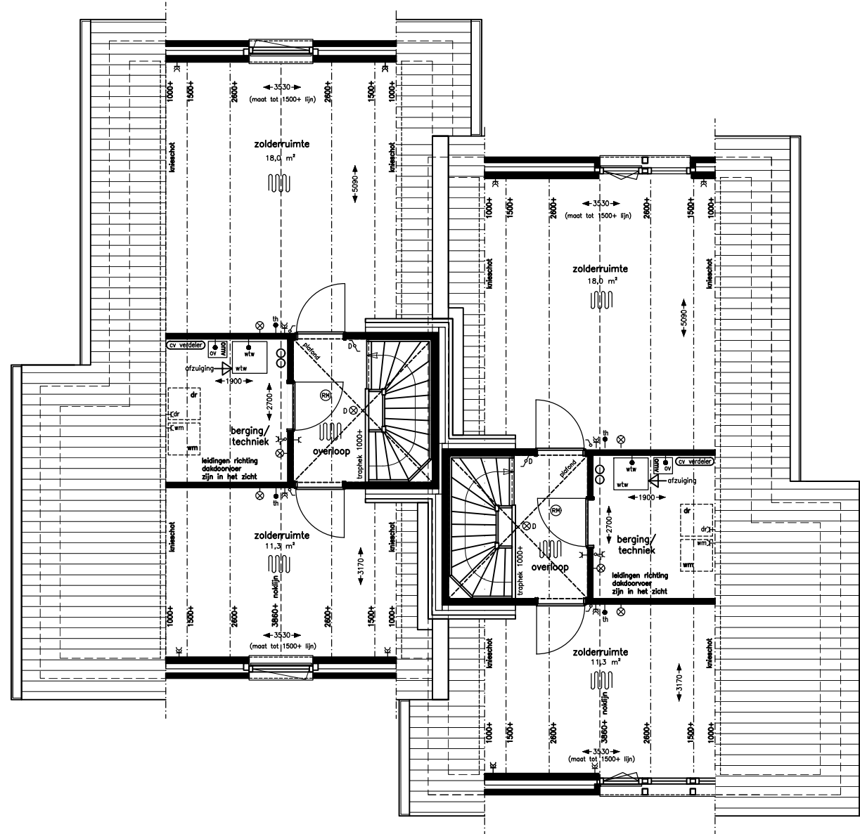
2e verdieping type B-P10 schaal 1:50
