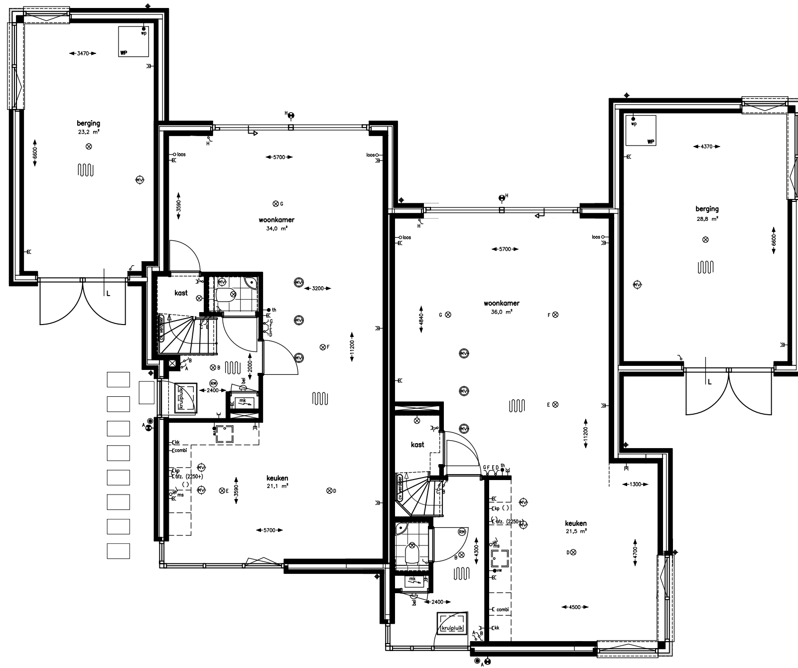
begane grond type A-P07 schaal 1:50
