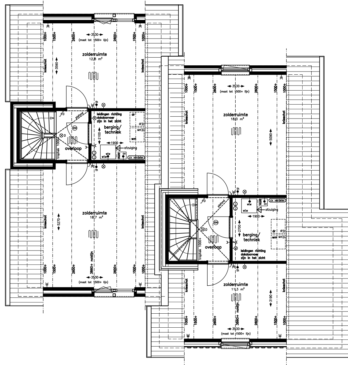
2e verdieping type A-P07 schaal 1:50
