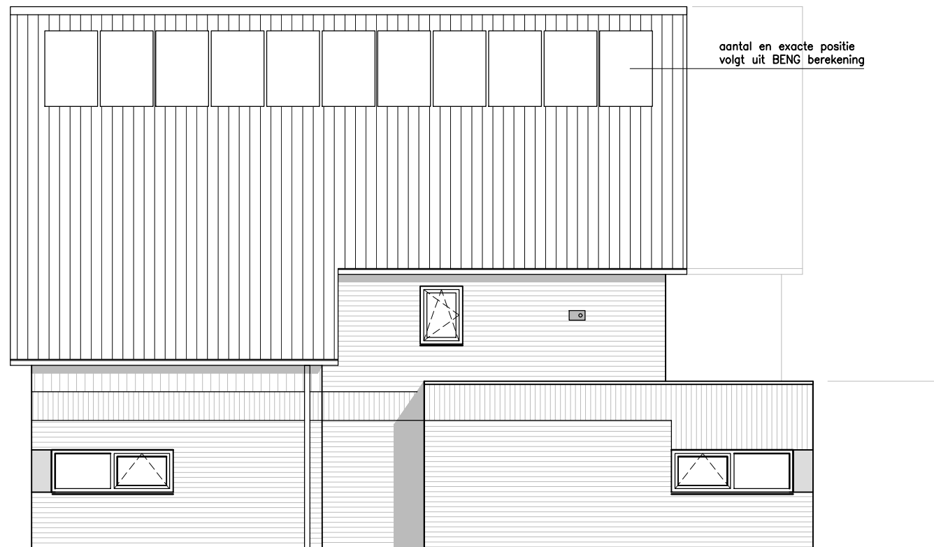
rechter zijgevel type B-P06 schaal 1:50
